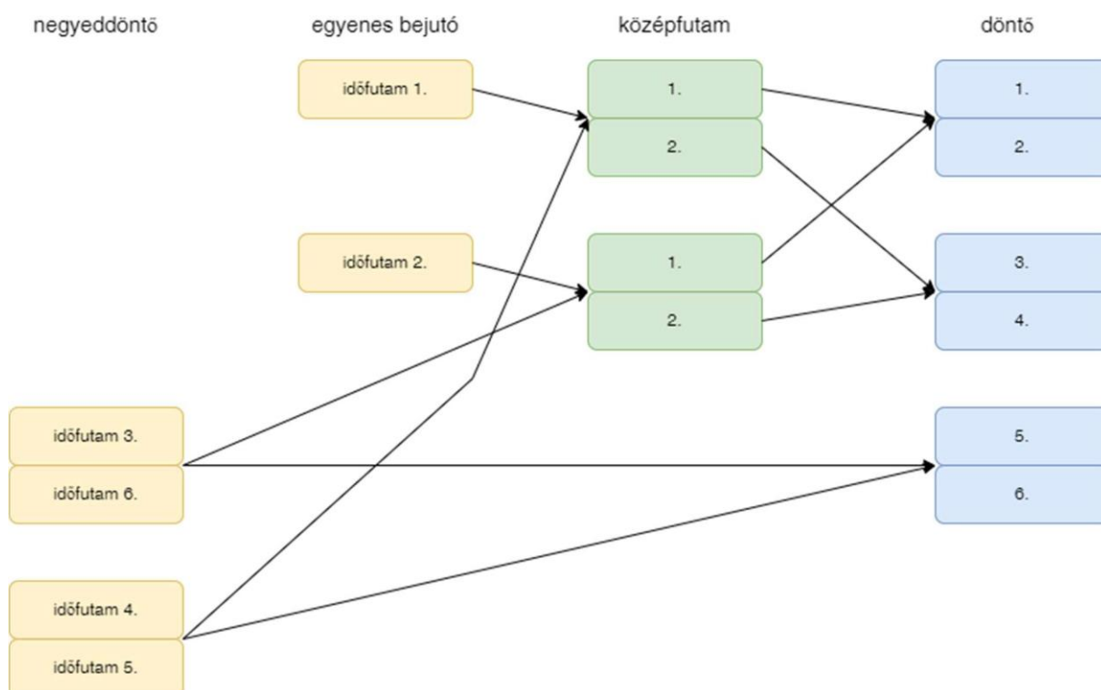
6. ábra: Továbbjutási rendszer 6 induló esetén az ifjúsági a felnőtt számokban
