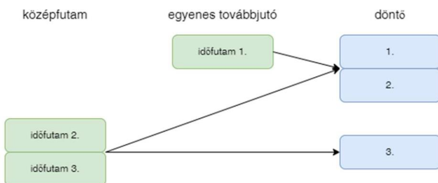
10. ábra: : Továbbjutási rendszer 3 induló esetén
