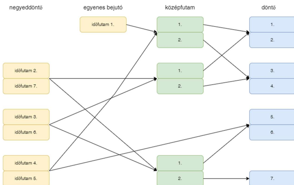
4. ábra: Továbbjutási rendszer 7 induló esetén az ifjúsági a felnőtt számokban
