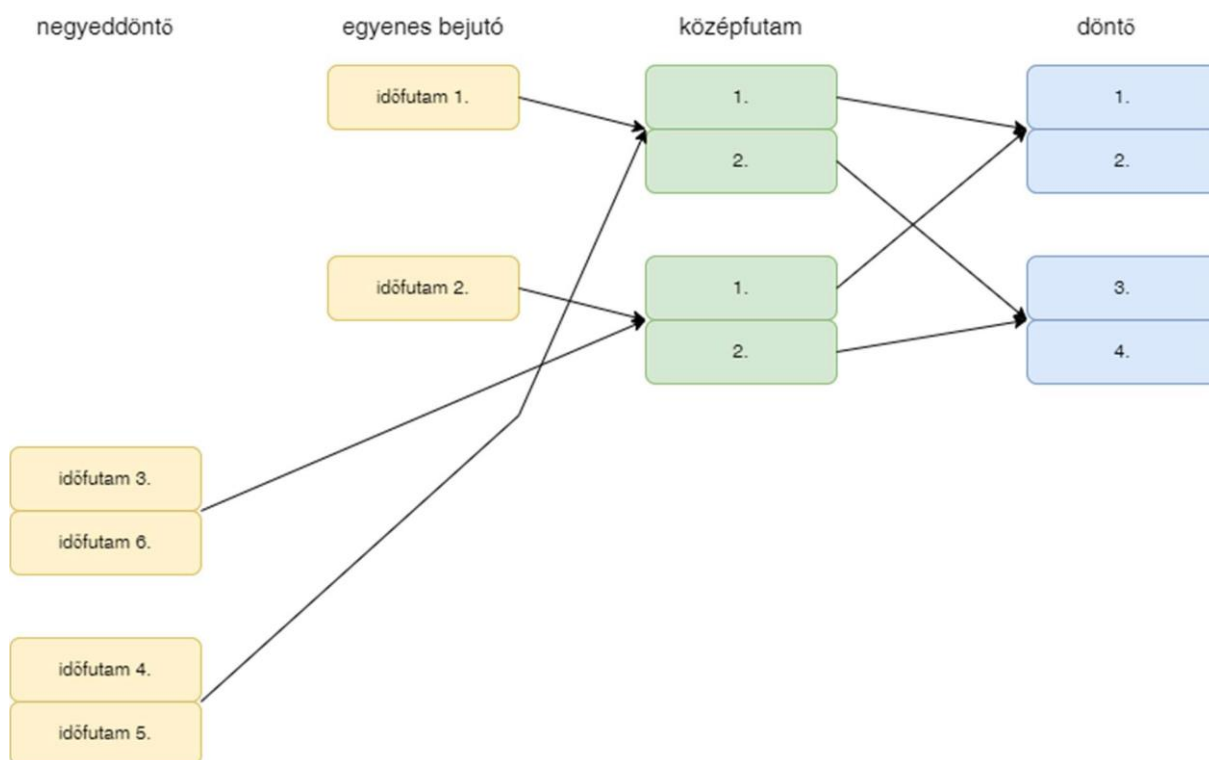
5. ábra: Továbbjutási rendszer 6 induló esetén az ifjúsági a felnőtt számokon kívül
