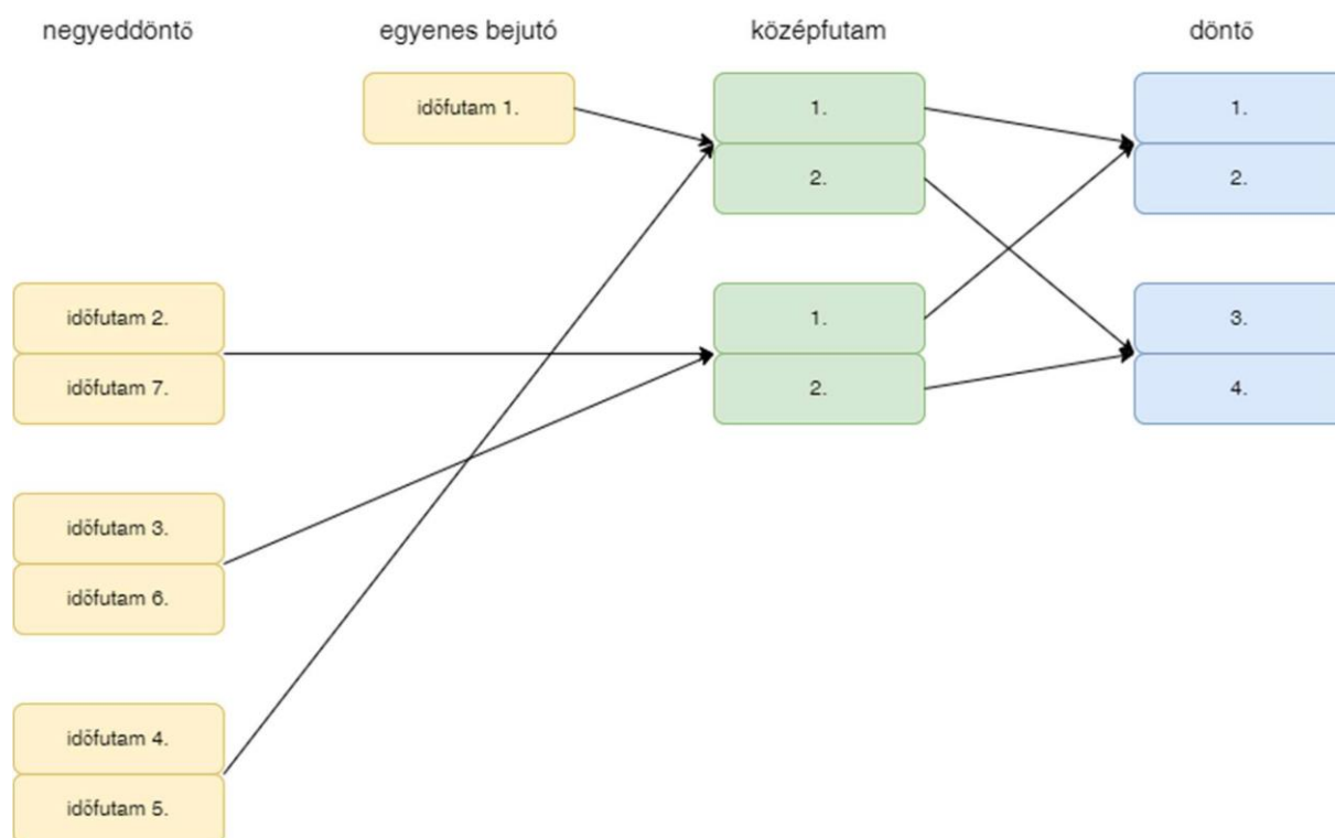
3. ábra: Továbbjutási rendszer 7 induló esetén az ifjúsági a felnőtt számokon kívül
